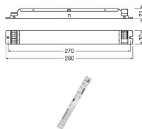
Scheda tecnica Osram LED Driver Optotronic Intelligent Dali Dimmerabile 1A0 NFC L
